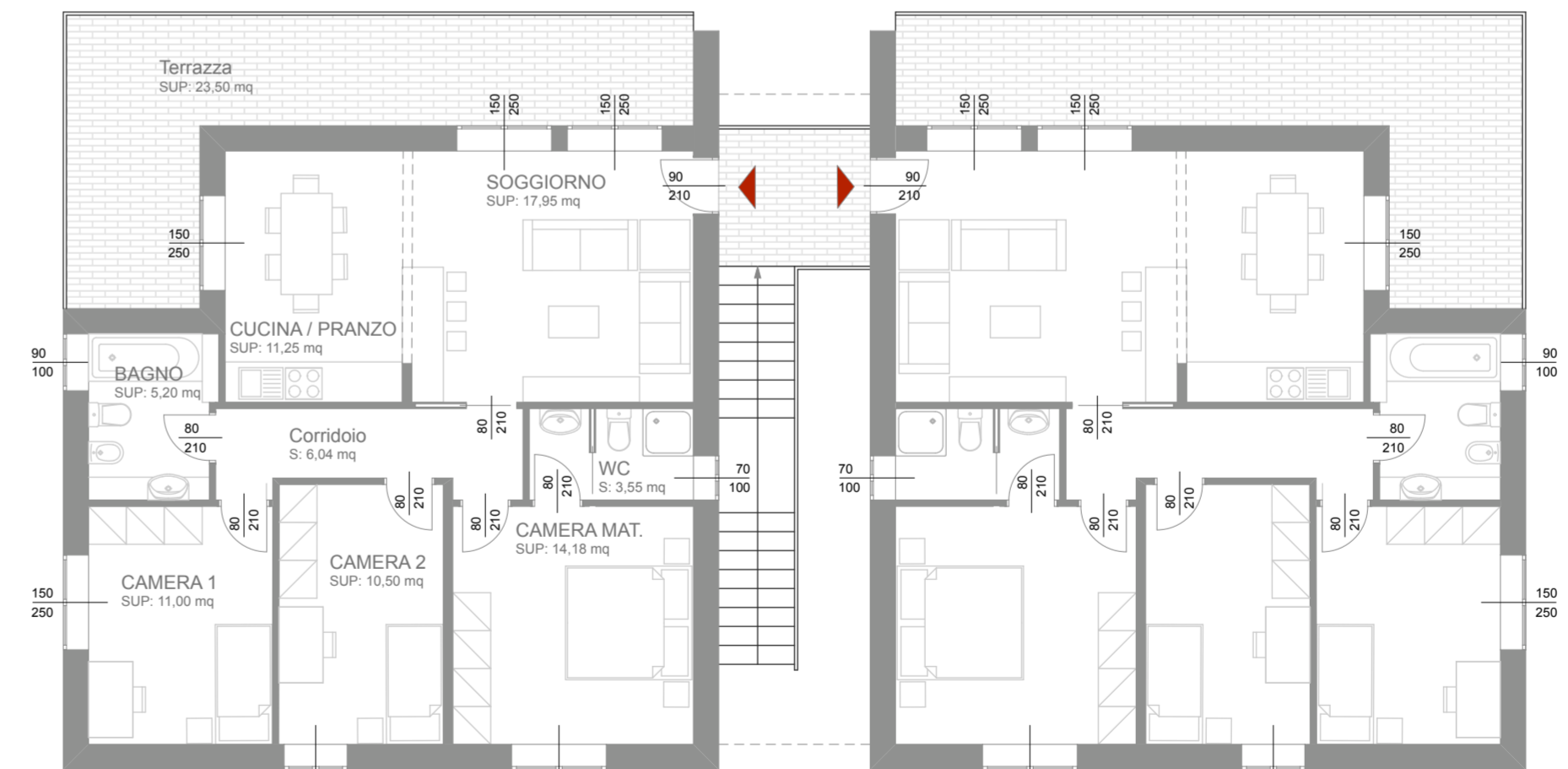
PIANO PRIMO_PALAZZINA_QUADRILOCALI
