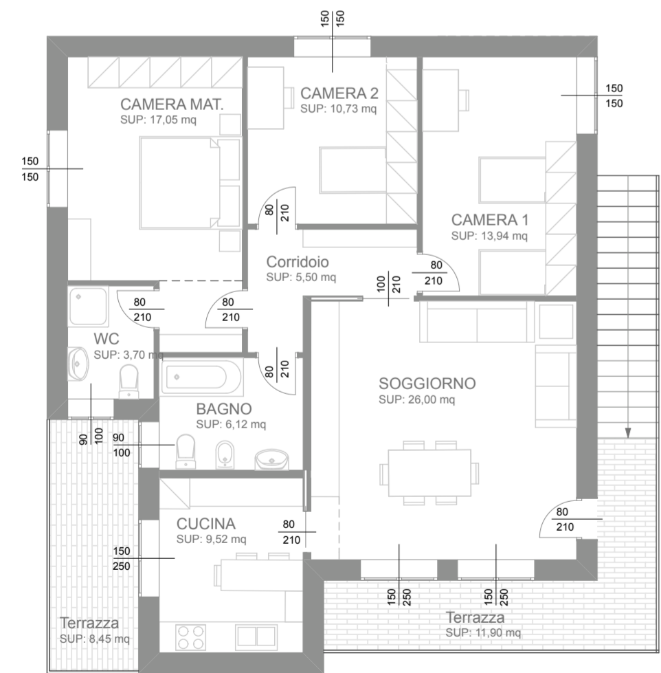
PIANO PRIMO_BIFAMILIARE_QUADRILOCALE
