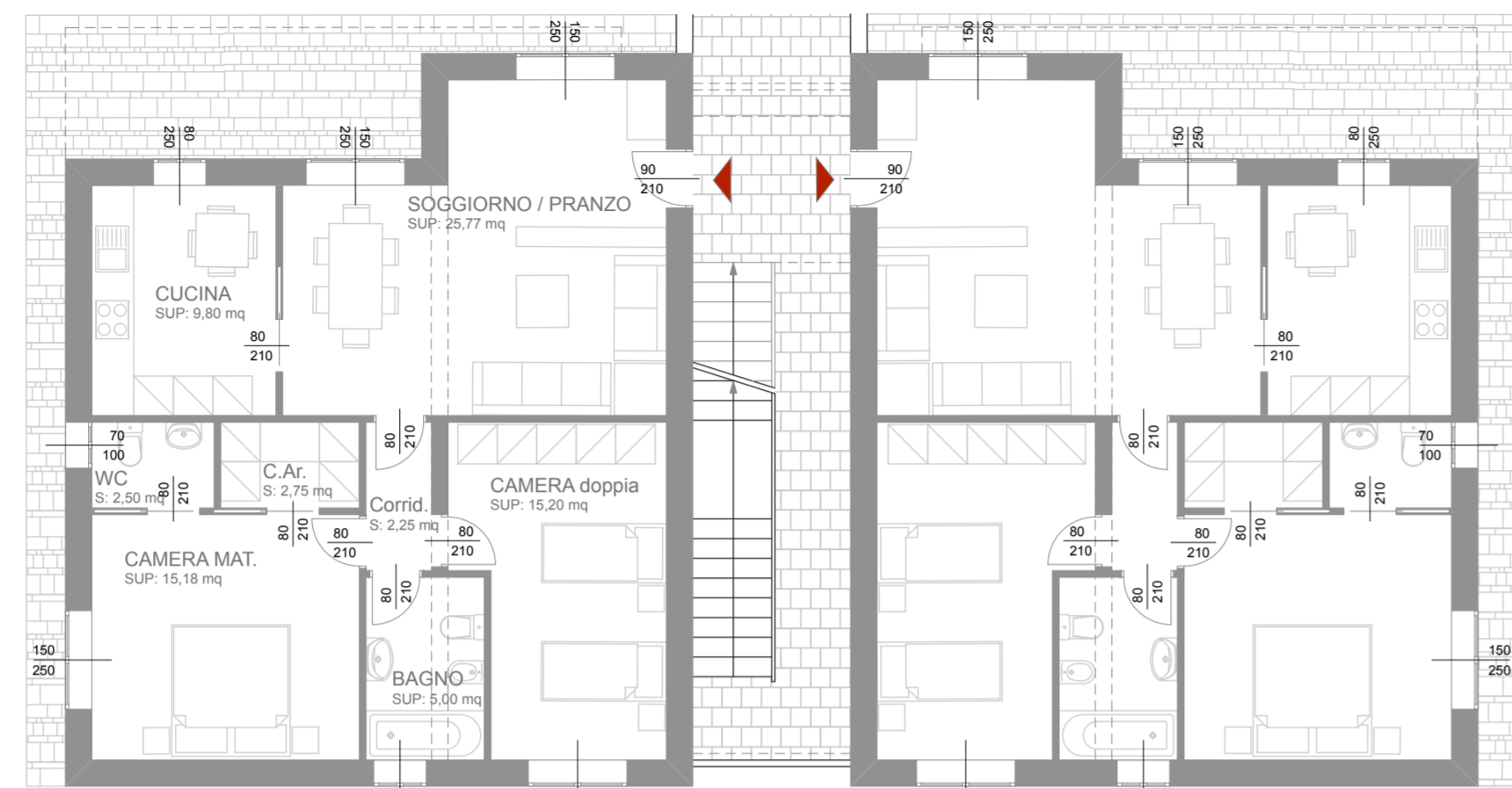
PIANO TERRA_PALAZZINA_TRILOCALI
