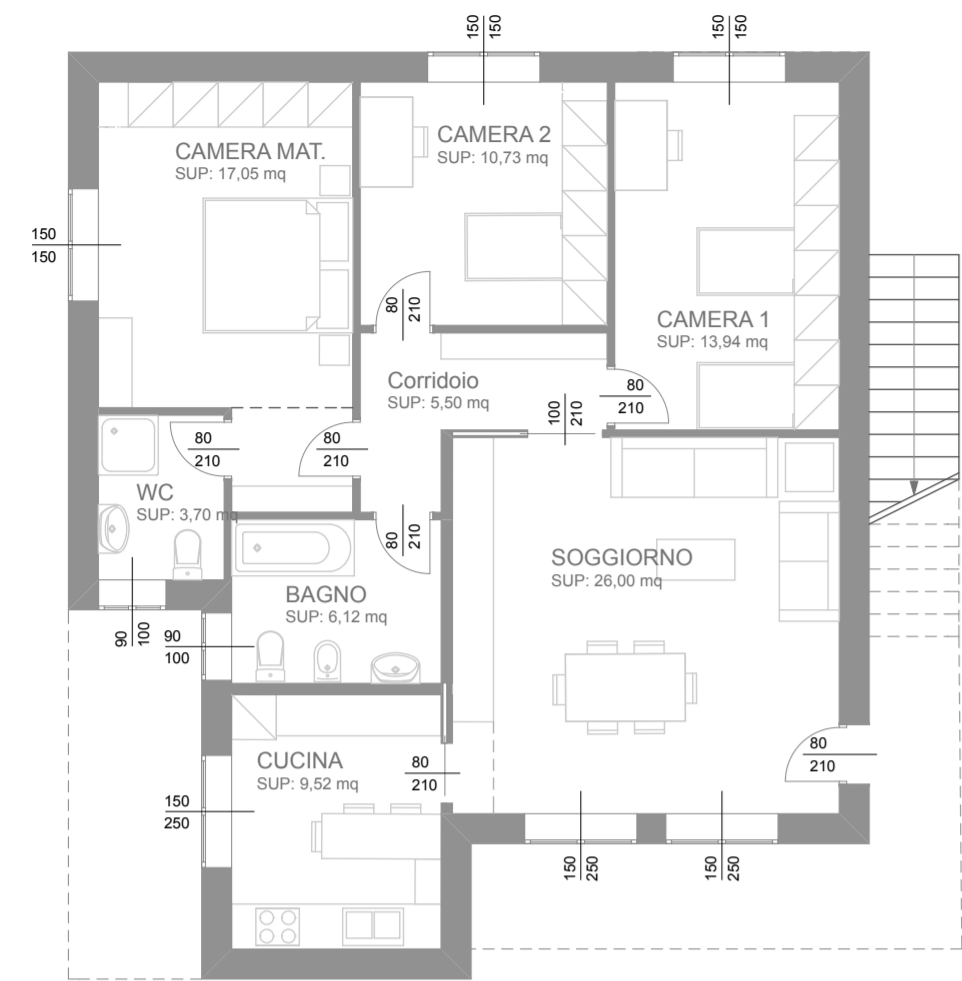
PIANO TERRA_BIFAMILIARE_QUADRILOCALE
